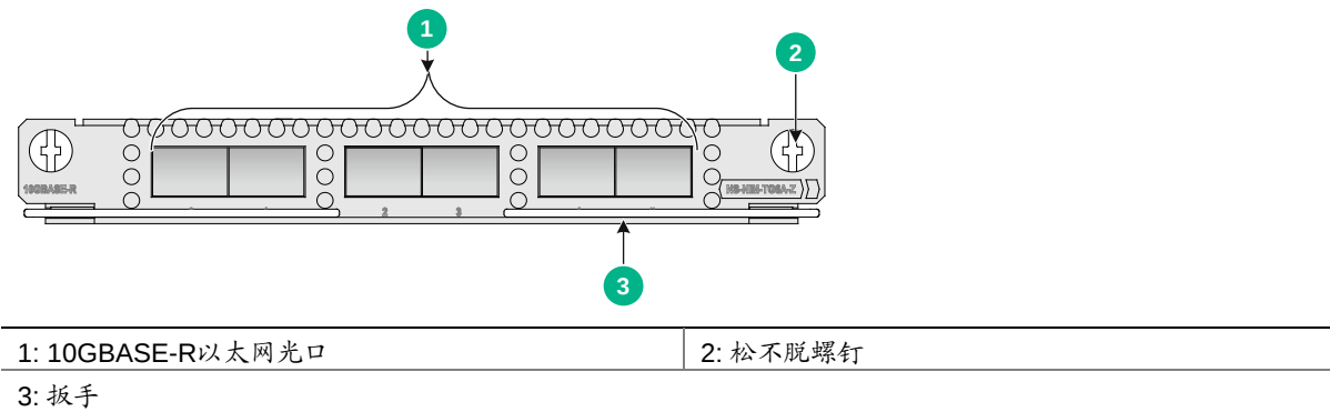
图A-7 NS-NIM-TG6A-Z 接口模块正视图
