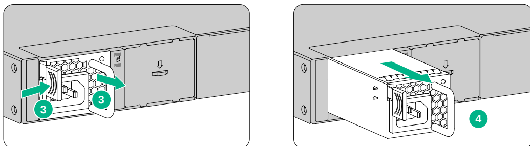
图4-2 拆卸电源模块
