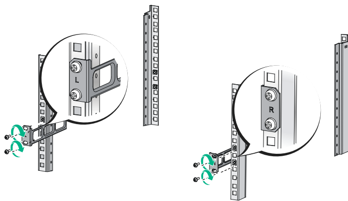
图2-3 安装后挂耳
