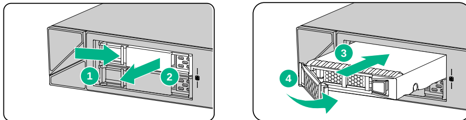
图2-12 安装硬盘
