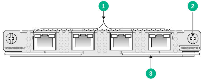
图A-5 NSQM1GT4PFC 接口模块正视图
