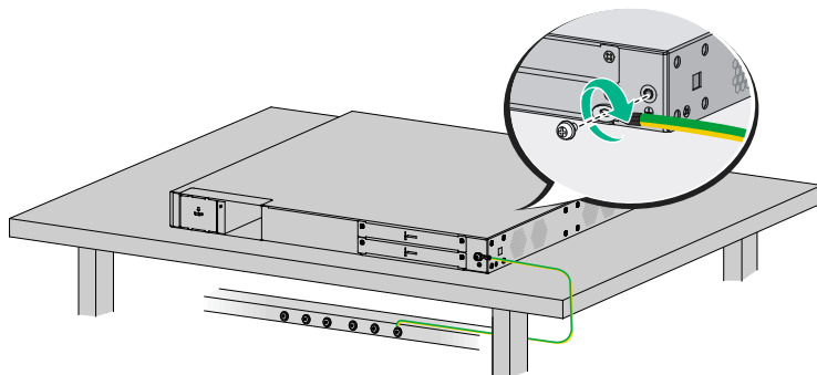
图2-6 通过接地排接地
