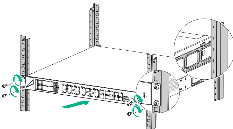
图2-5 安装设备到机柜
