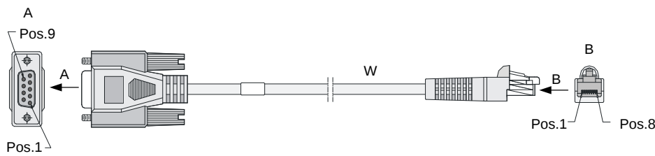
图C-1 CONSOLE 口和 PC 机（或终端）的串口之间电缆示意图。
