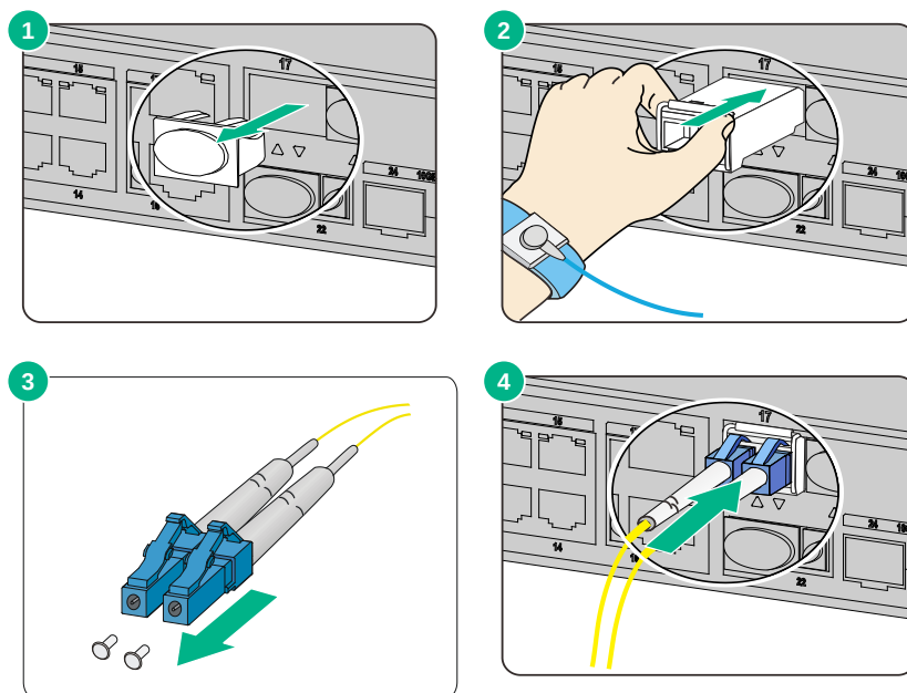
图2-16 安装及连接光模块
