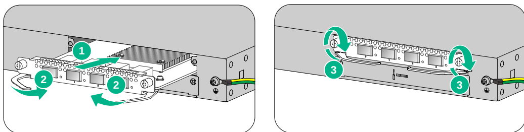
图2-11 安装接口模块
