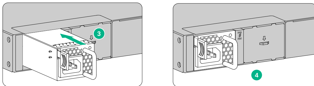
图2-9 安装电源模块
