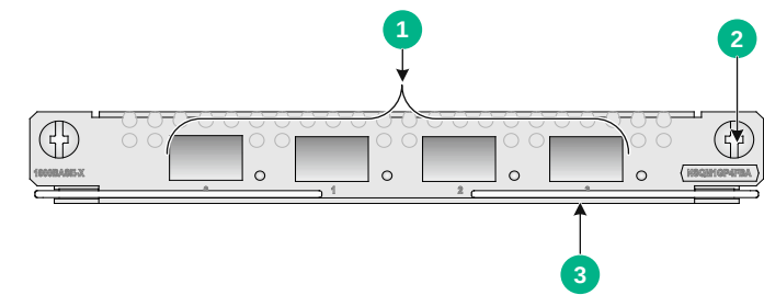
图A-6 NSQM1GP4FBA 接口模块正视图
