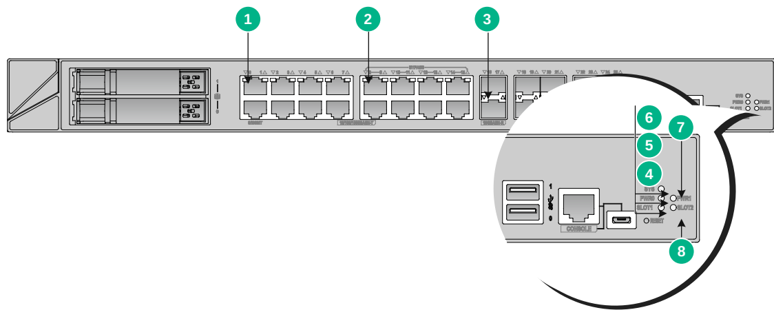
图B-1 T1000-CN80 指示灯
