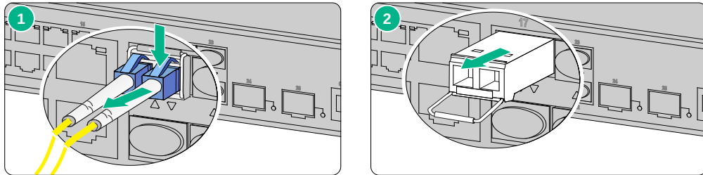
图4-5 拆卸光接口模块示意图
