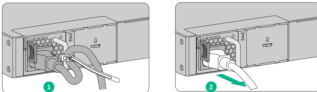
图4-1 拆卸电源模块
