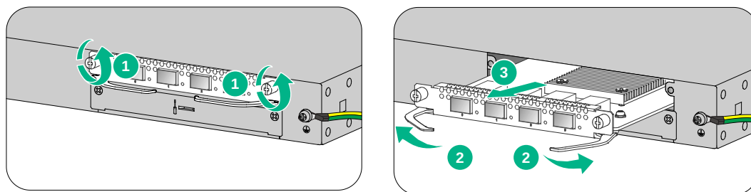
图4-3 拆卸接口模块
