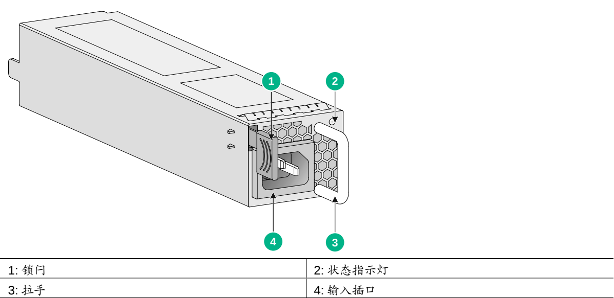
图A-8 PSR250-12A1-Z 交流电源模块外观
