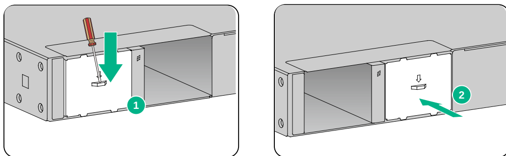
图2-8 拆卸电源假面板
