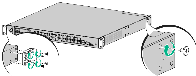
图2-4 安装前挂耳和承重螺钉
