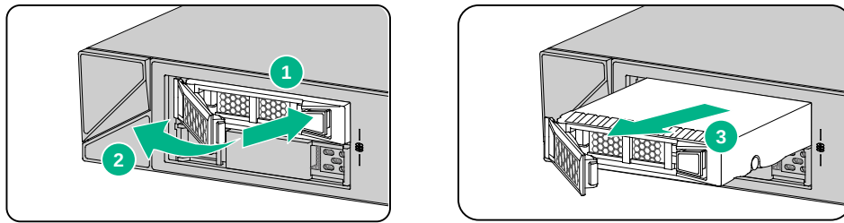
图2-13 拆卸硬盘
