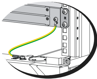
图2-7 连接到机柜接地
